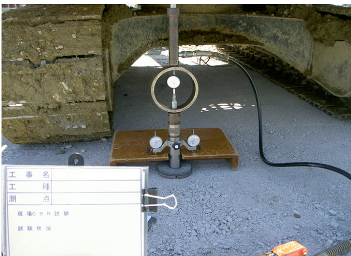
現場CBR試験 (JIS A 1222)
